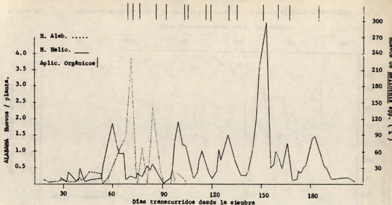
FIGURA No. 14 Representación gráfica de las poblaciones de huevos de Alabama argillacea - vs - huevos de Heliothis spp., Lote 12, año 1978
